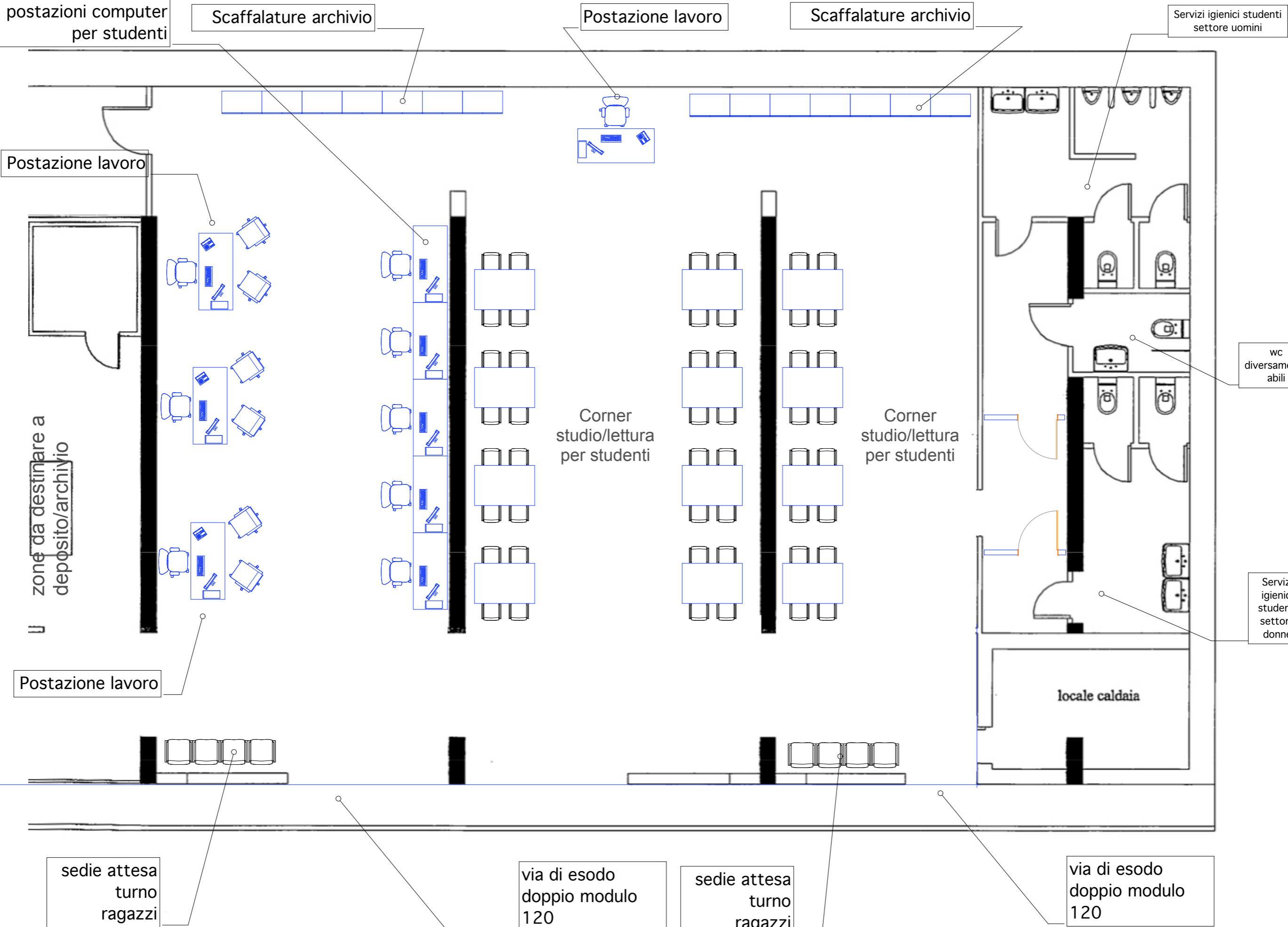
PLANIMETRIA PARTICOLARE PROPOSTA ALLESTIMENTO ZONA APERTA AL PUBBLICO
